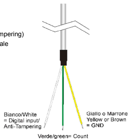
Fig. 12 – Terminazione cavo di conteggio
