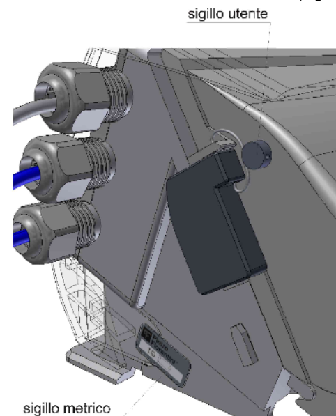
Fig. 10 – Sigilli metrici ed utente
